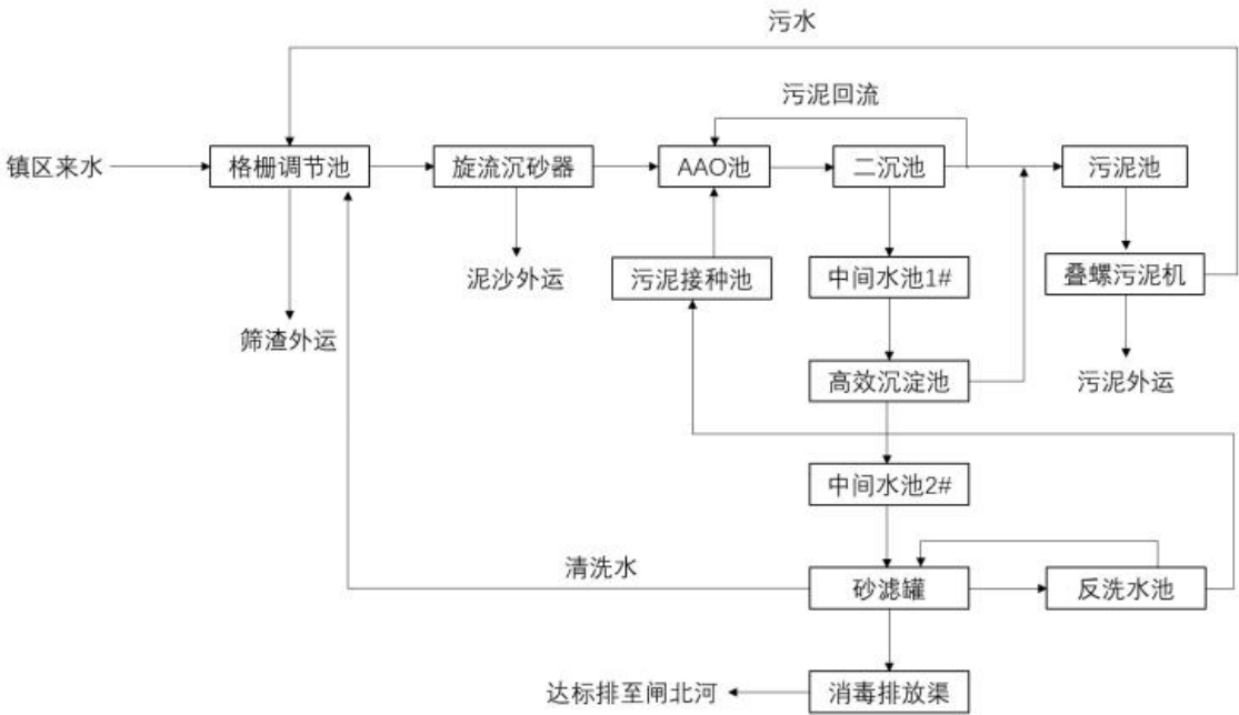
图 2-4 工艺流程示意图
