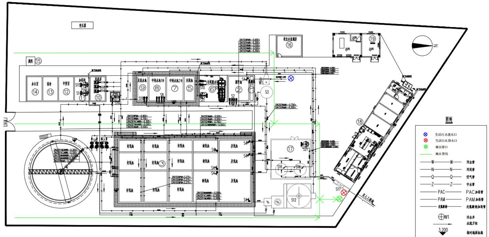
图 2-2 本项目平面布置图
