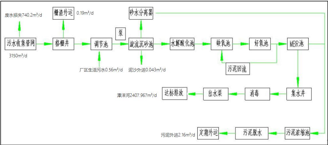
图 2-3 本项目水平衡图
