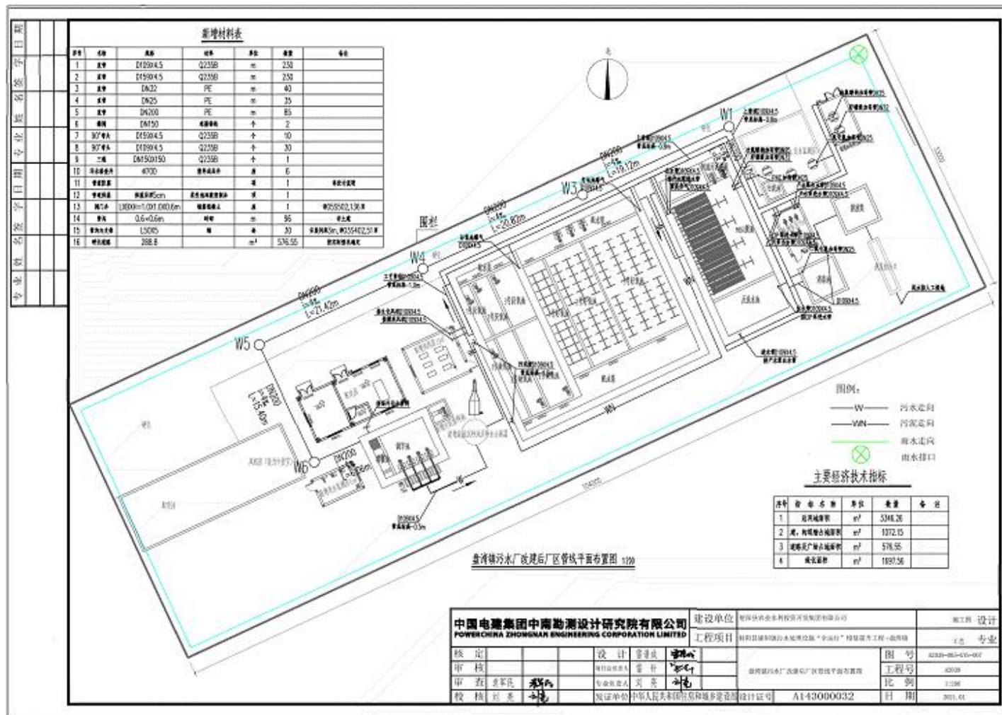
图 2-2 本项目平面布置图
