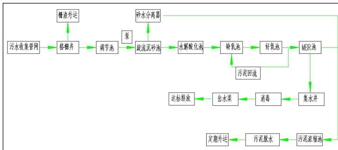
图 2-4 工艺流程示意图
