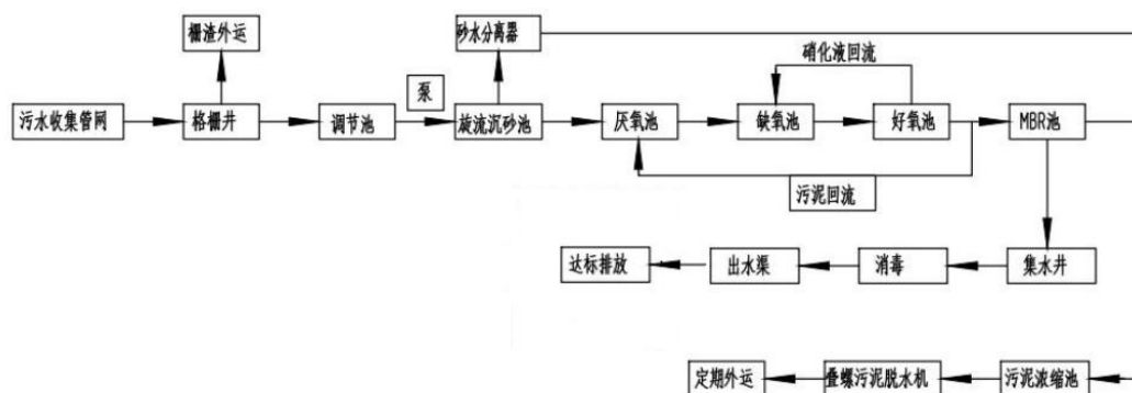
图 2-4 工艺流程示意图
