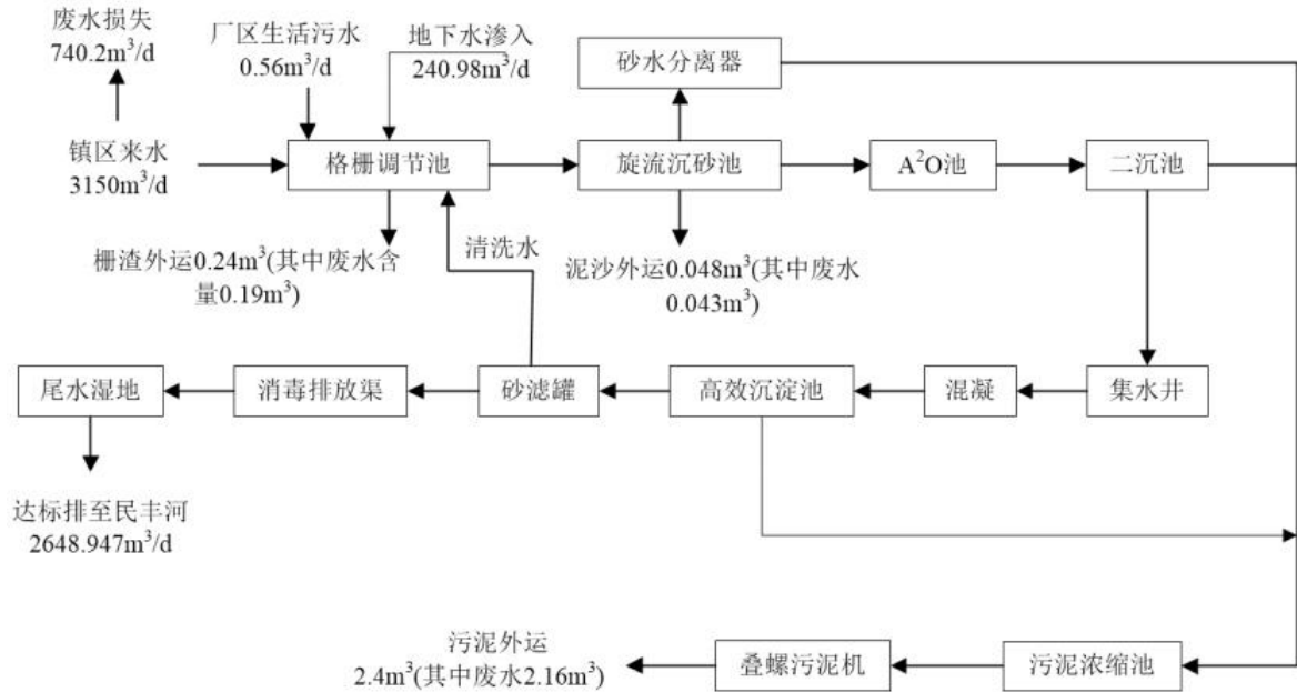
图 2-4 工艺流程示意图
